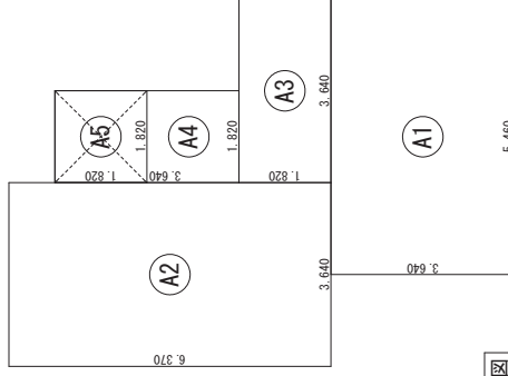
2階 床面積求積図
