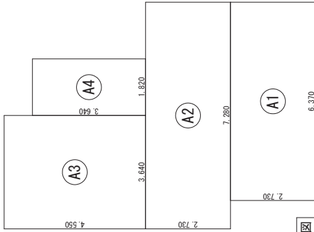
1階 床面積求積図
