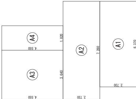
建築面積求積図
