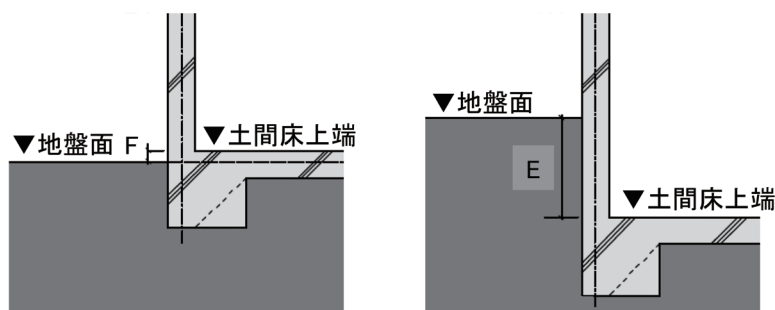
土間床上端が地盤面と同じか高い場合 土間床上端が地盤面よりも低い場合
