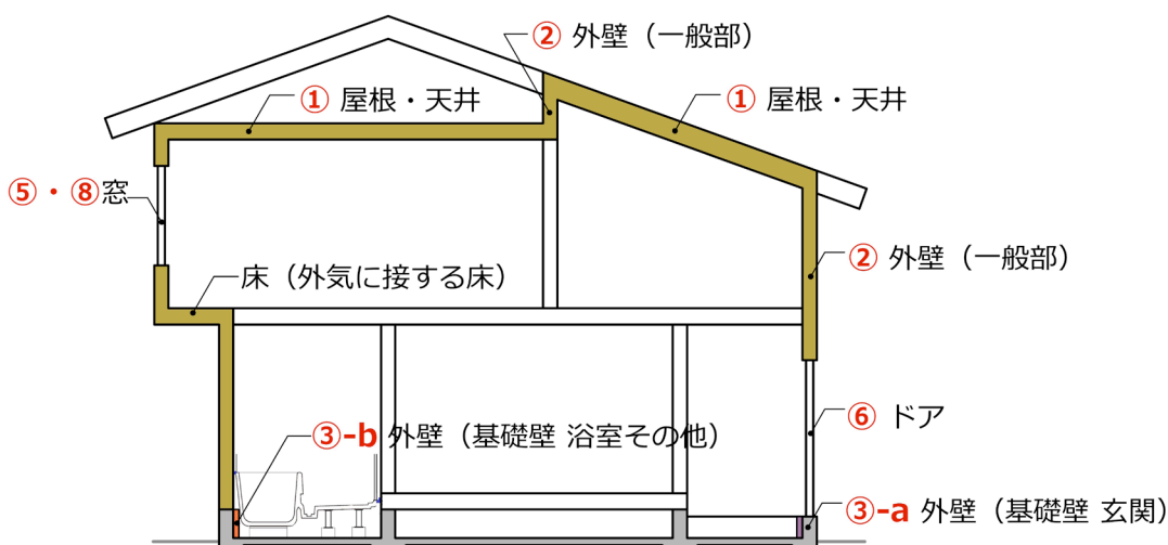
—断面図—
