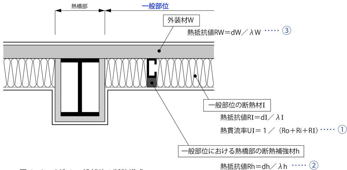
図 4. 2 S 造の一般部位の断熱構成
